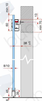
Регулировка в трех плоскостях
