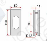
34.7007.99 Ручка для стекла 10–12 мм
