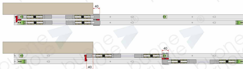
58.8325.22 Фиксатор неподвижного стекла
