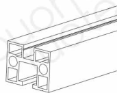
Горизонтальный профиль 11.1024.03/N — черный 11.1024.03/B — белый 11.1024.03/G — под окраску
