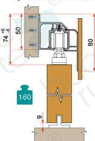
Крепление к стене
