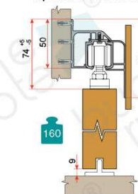
Крепление к стене
