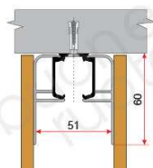
Держатель декора- тивного профиля 42.8325.02/50/G - al
