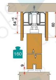
Раздвижная перегородка
