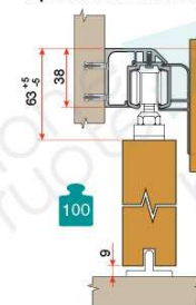
Крепление к стене ЭКО
