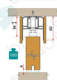
Крепление к потолку
