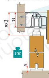
Крепление к стене ЭКО
