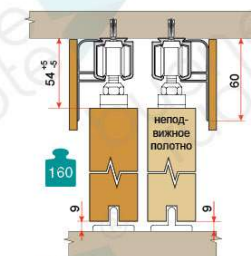
Раздвижная перегородка с неподжным полотном
